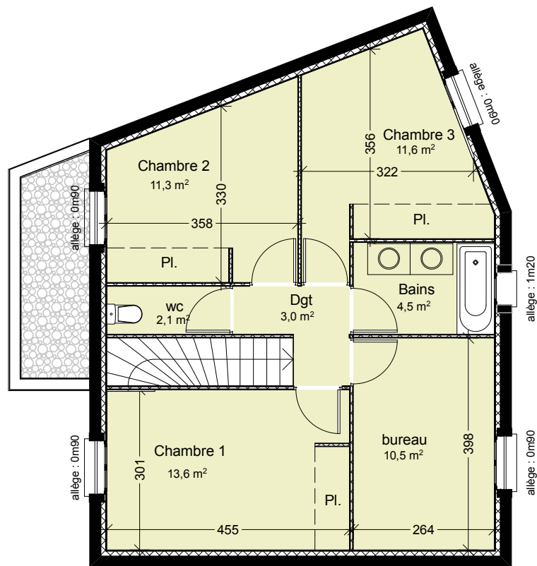
MAISON DE VILLE NIVEAU 1 / T5 Lot 1
